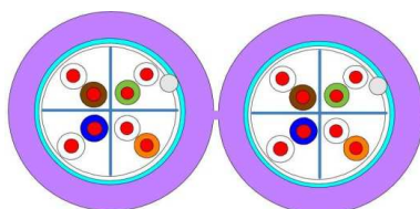
Rys. Kabel skrętkowy typu duplex
